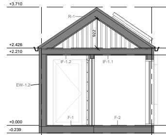
SECTION A-B M 1 : 50
