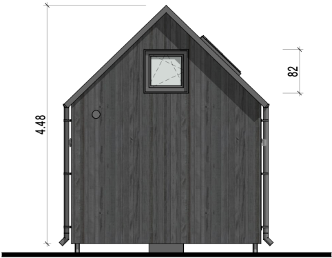
F2 ELEVATION 1:75
